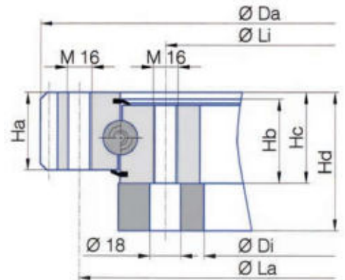
SEZ. B-B
